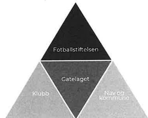
Figur 5-1: Gatelagens samarbeidsmodell
