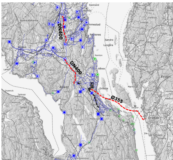
Figur 26: Tiltakspakke Alt L1 - Overføring Heggedal - Åsgård + L0
