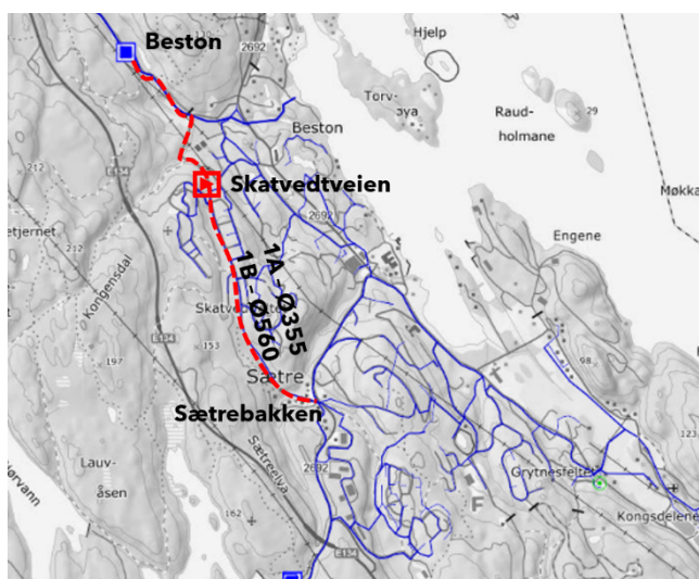
Figur 20: Tiltakspakke Alt 1-Skatvedt
