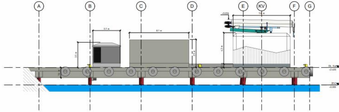
1 Fasade Nord-Vest 1 : 100
