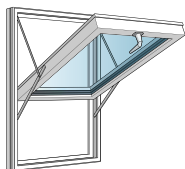
TSG 180 Horisontellt glidhängt 180° öppning
