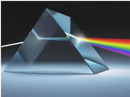
الضوء بعد مروره من منشور زجاجي
