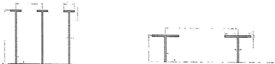
Slika 6.1. Detalji obilježavanja upravnog parking mjesta; Slika 6.2 Detalj obilježavanja podužnog parking mjesta
