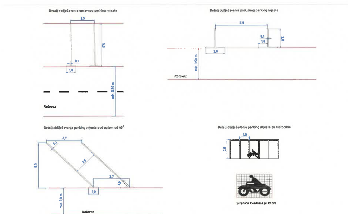
Slika 5.1 Detalj obilježavanja parking mjesta za putničke automobile i motocikle
