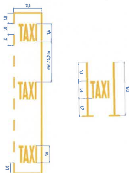
Slika 5.3 Detalj obilježavanja taxi stajališta
