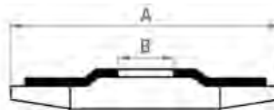
Type G 27 (conical 8°)
