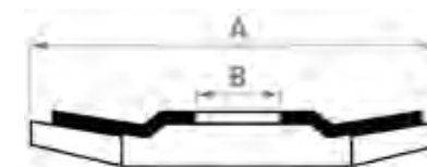
Type G 19 (conical 15°)
