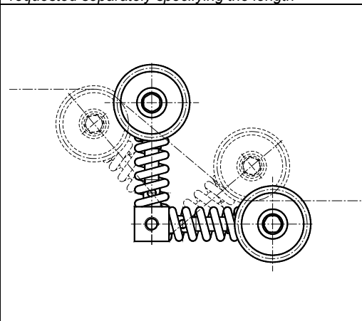
Fig.9 Doppia tensione con "angolo V" per doppio recupero. Double tensioner with "V angle" for double recovery
