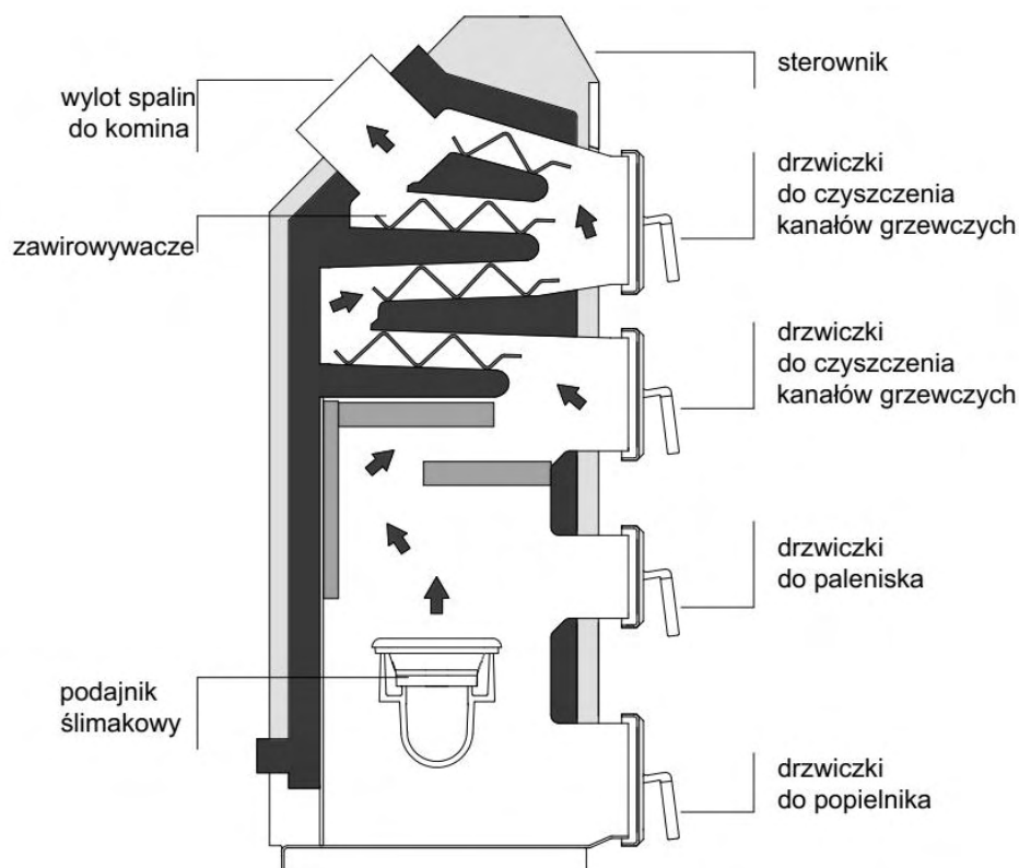
Rys 1. Przekrój kotła
