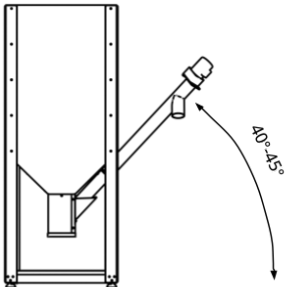
Rys. 17 - Ustawienie rury podajnika zewnętrznego
