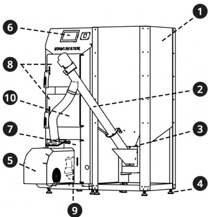
Rys. 1 - Elementy z przodu kotła (10kW)
