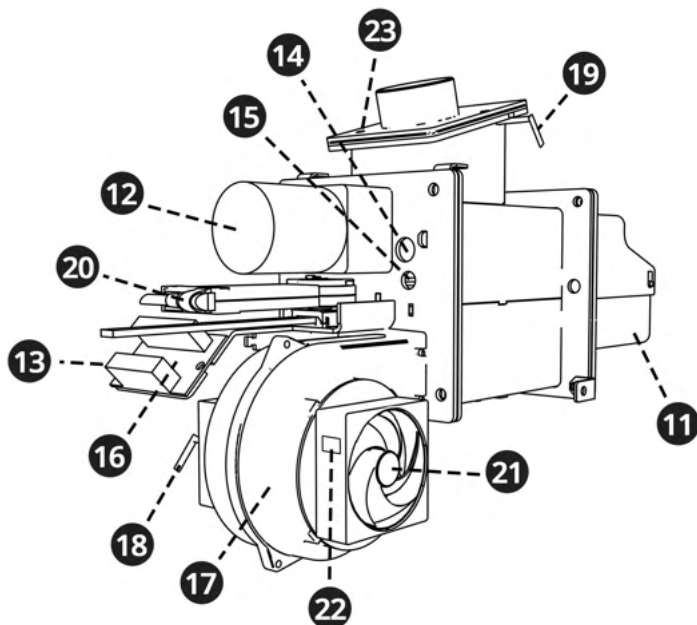
Rys. 14 - Tył palnika
