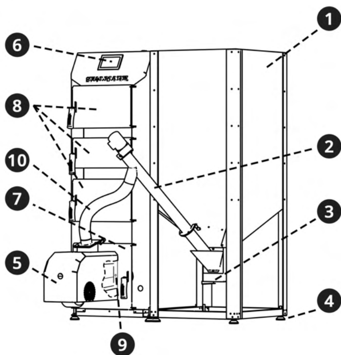
Rys. 9 - Elementy z przodu kotła (25-35kW)
