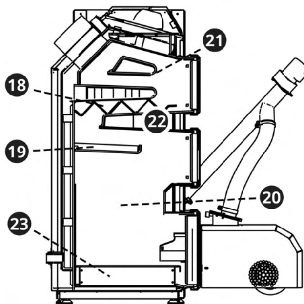
Rys. 4 - Elementy wewnątrz kotła (10kW)
