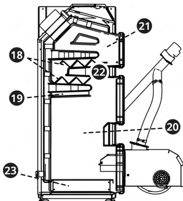
Rys. 8 - Elementy wewnątrz kotła (15-20kW)
