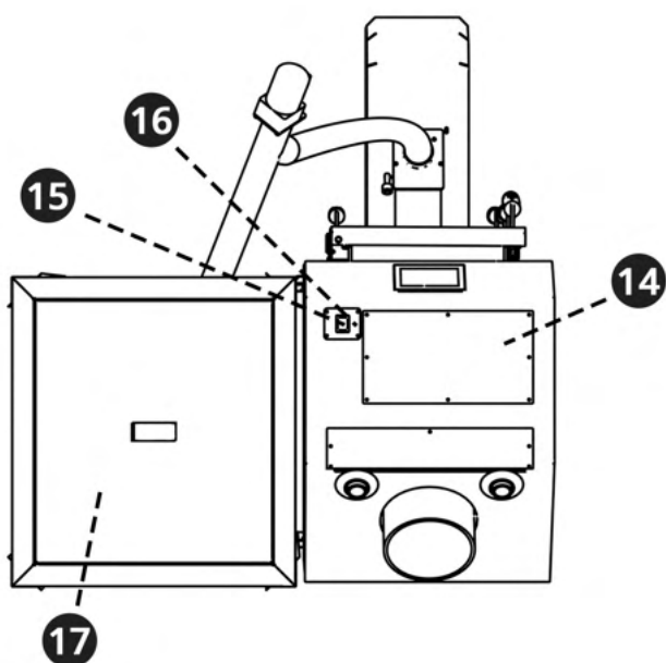
Rys. 11 - Elementy na górze kotła (25-35kW)
