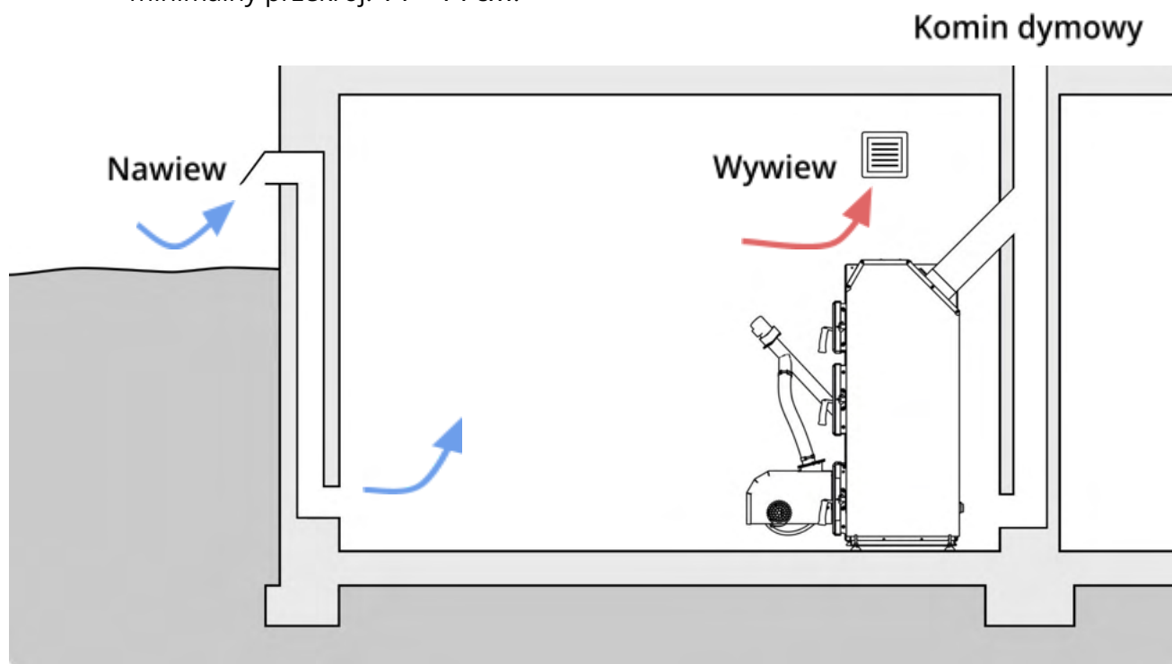
Rys. 17 - Umiejscowienie elementów wentylacji
