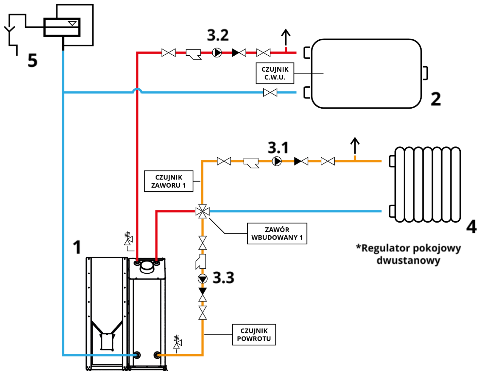
Rys. 18 - Układ otwarty z zaworem czterodrogowym
