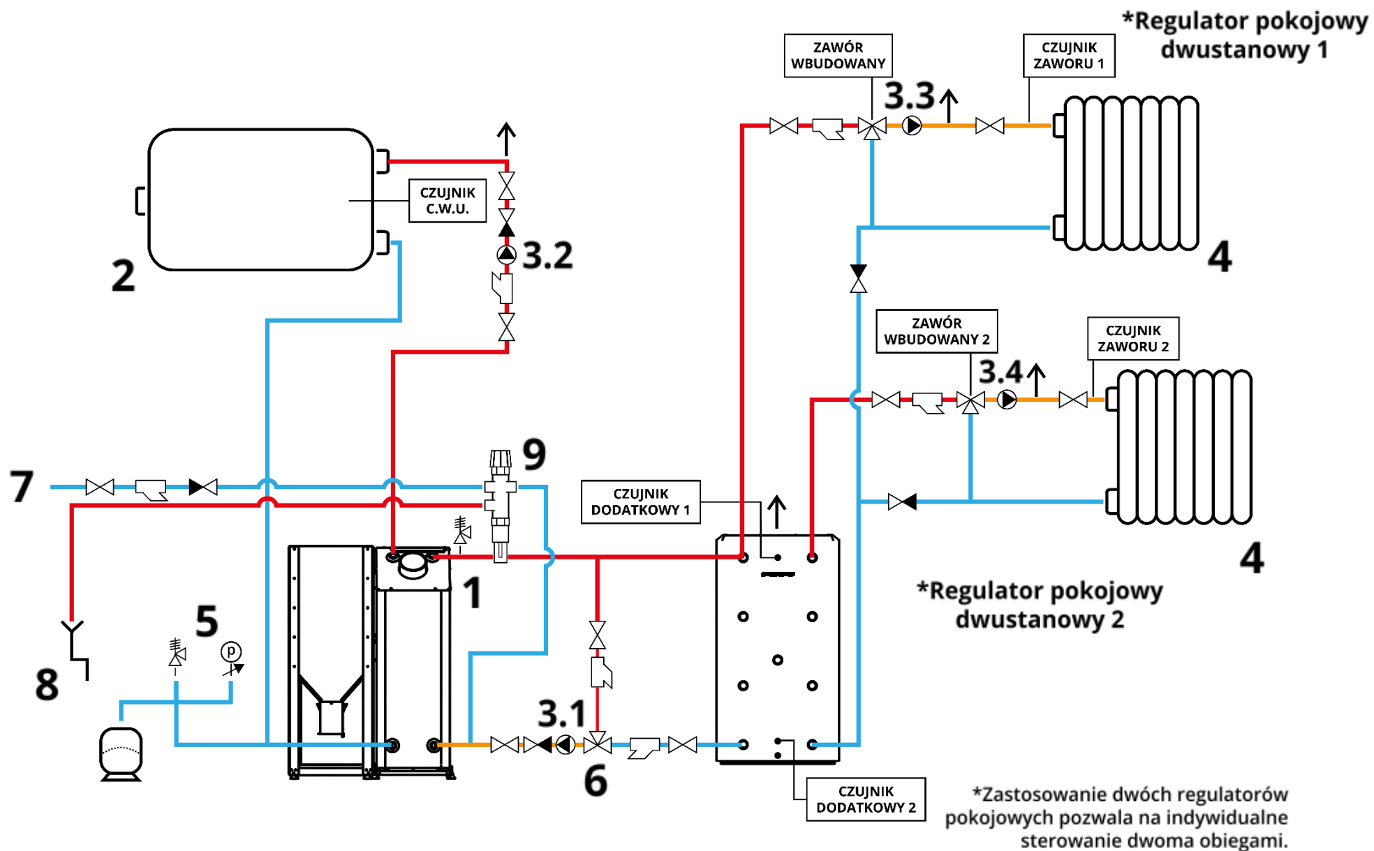
Rys. 20 - Układ zamknięty z buforem i zaworem termostaticznym
