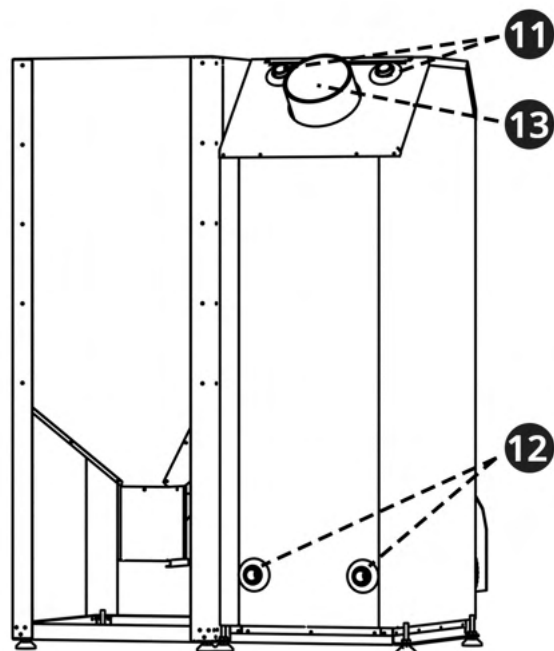
Rys. 10 - Elementy z tyłu kotła (25-35kW)
