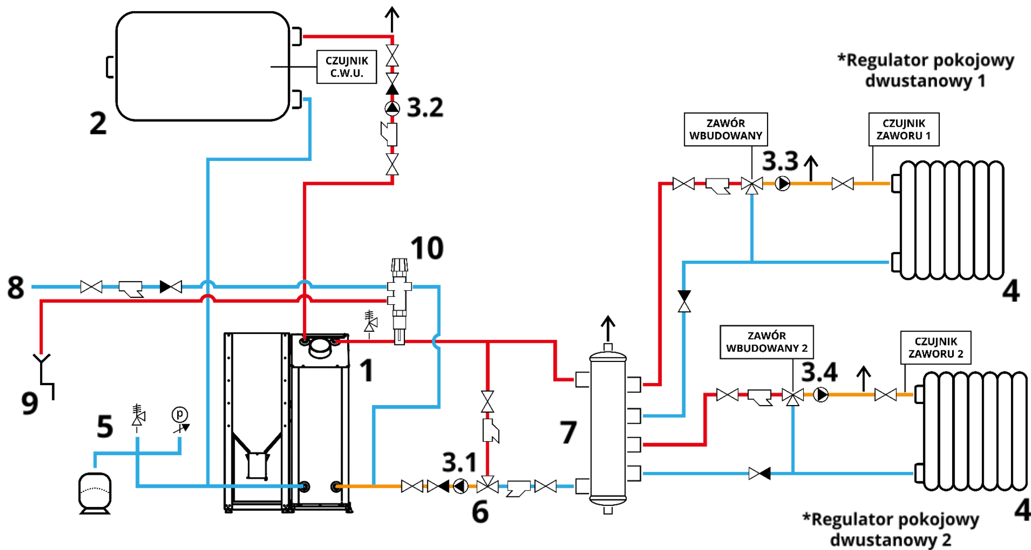
Rys. 22 - Układ zamknięty ze sprzęgłem i zaworem termostaticznym
